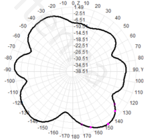
960.0MHz Total(E2-YZ), Max= 1.09dBi
