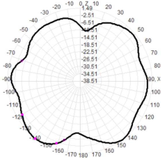
960.0MHz Total(E1-XZ), Max= 1.49dBi
