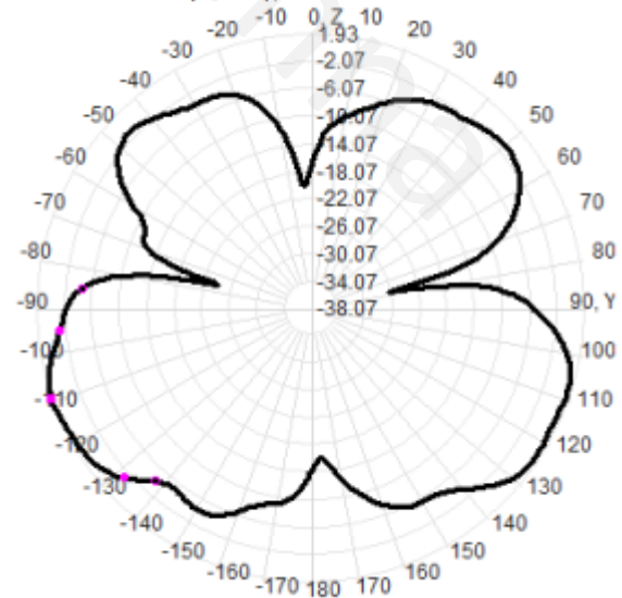
2300.0MHz Total(E2-YZ), Max= 1.92dBi
