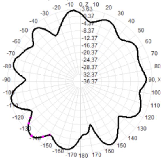
2400.0MHz Total(E1-XZ), Max= 3.63dBi
