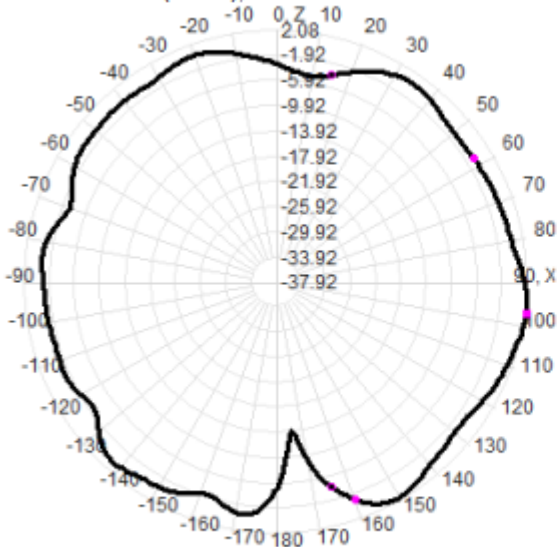
2710.0MHz Total(E1-XZ), Max= 2.08dBi
