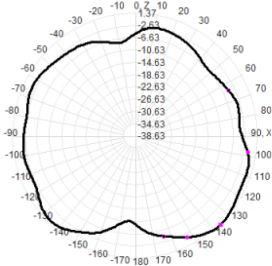
960.0MHz Total(E1-XZ), Max= 1.37dBi
